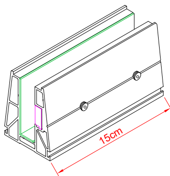
سانتی شیشه گیر 15 پک ماشین کاری شده با پراق inner glazing gasket
