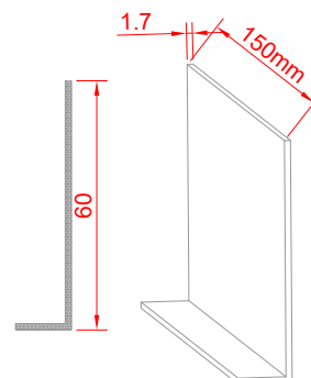
code : 2000-137 نصب شیشه GLAZING WEDGE
