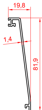
code :21386 پروفیل کاور شیشه گیر cover profile weight : 0.446 kg/m
