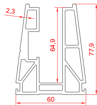
code :21385 پروفیل شیشه گیر Glass support base shoe weight : 3.24 kg/m
