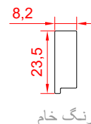
code :21387 پروفیل قفل شیشه pressing stick weight : 0.510 kg/m
