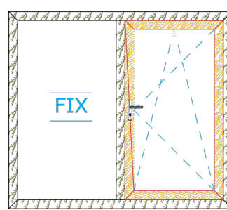
تک لنگه باز شو دو حالته
